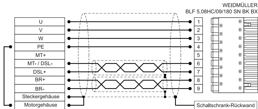
Abbildung 19: Steckerbelegung „Motor mit HIPERFACE DSL® [X6]“
