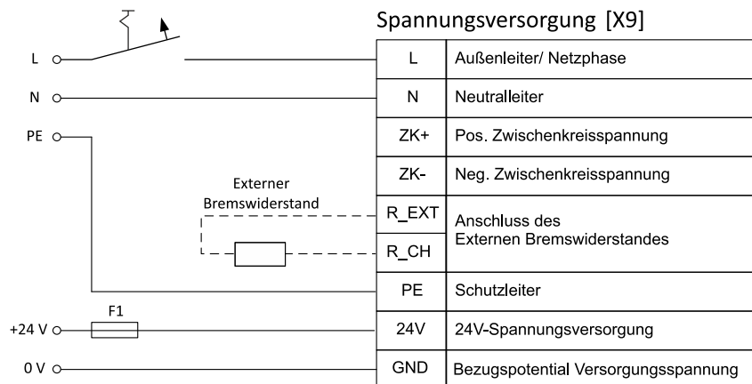
Abbildung 10: Anschluss eines BL 4102-C/BL 4104-C an die Versorgungsspannung [X9]
