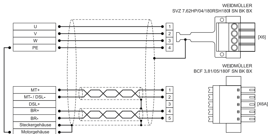
Abbildung 20: Steckerbelegung „Motor mit Motortemperatur-Sensor [X6], [X6A]“
