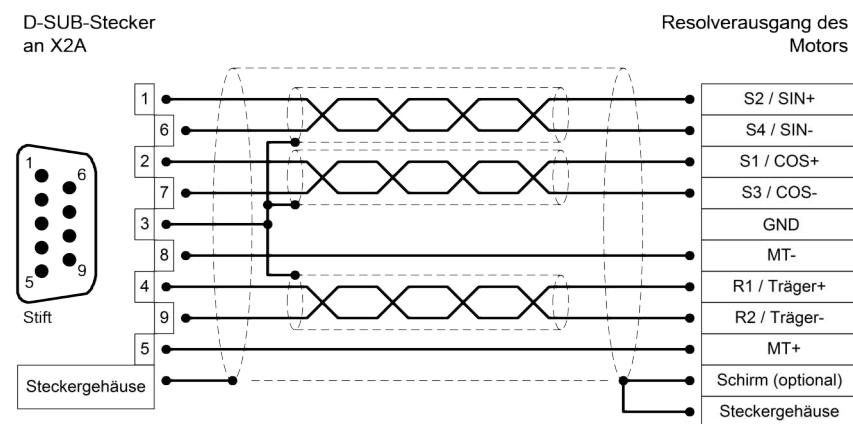
Abbildung 24: Steckerbelegung: Resolveranschluss [X2A]
