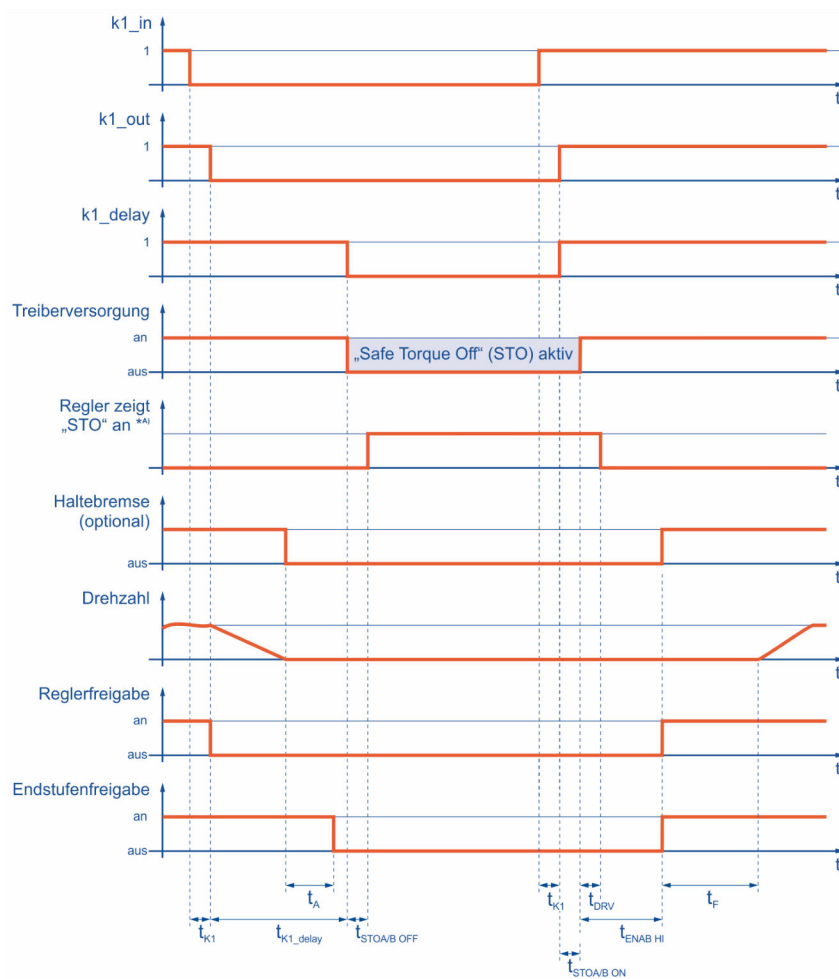
Abbildung 38: Zeitverhalten beim Aktivieren der Sicherheitsfunktion SS1 (externe Beschaltung) mit Wiederanlauf
