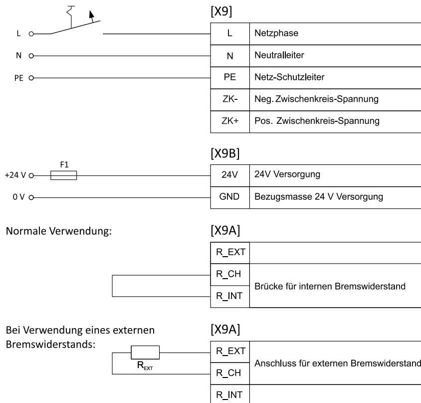
Abbildung 12: Anschluss eines BL 4108-C an die Versorgungsspannung [X9]
