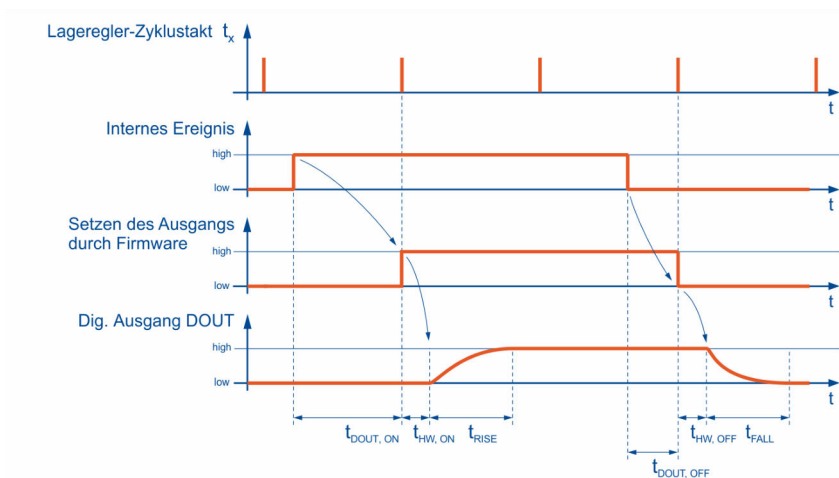
Abbildung 35: Mechanismus der Filterzeit bei digitalen Ausgängen
