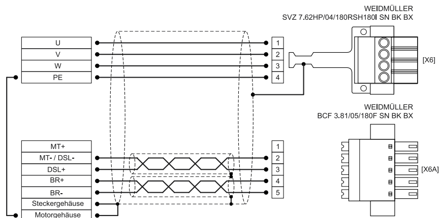
Abbildung 21: Steckerbelegung „Motor mit HIPERFACE DSL® [X6], [X6A]“
