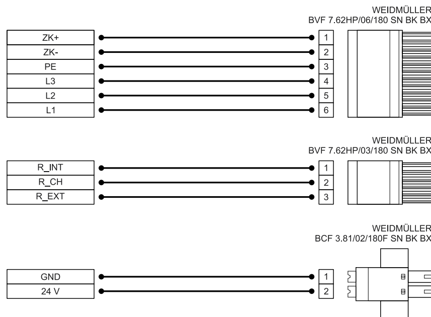
Abbildung 15: Steckerbelegung „Versorgungsspannung [X9], [X9A], [X9B]“
