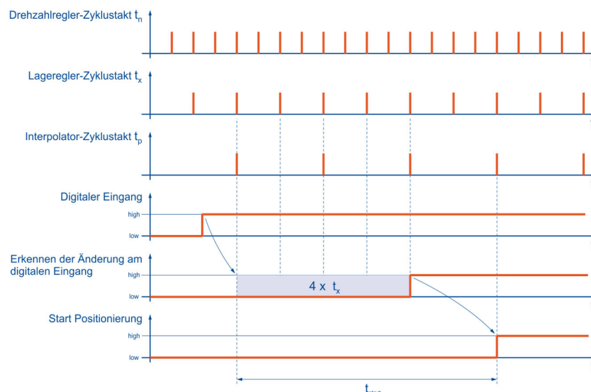
Abbildung 34: Mechanismus der Filterzeit bei digitalen Eingängen
