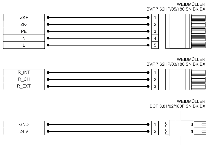
Abbildung 13: Steckerbelegung „Versorgungsspannung [X9], [X9A], [X9B]“
