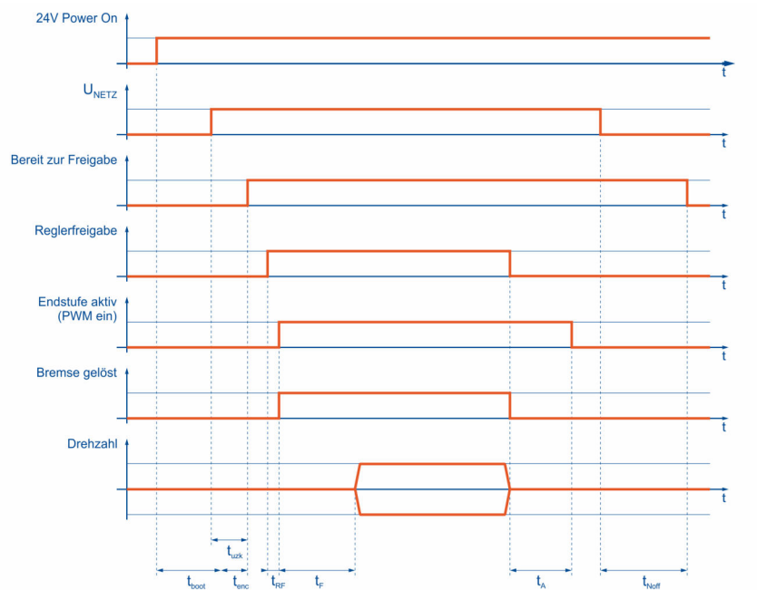
Abbildung 36: Timingdiagramm des Servoreglers
