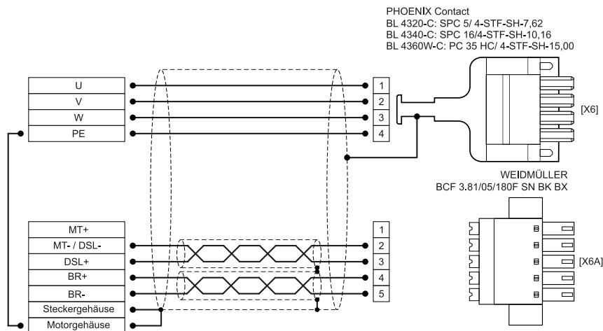
Abbildung 23: Steckerbelegung „Motor mit HIPERFACE DSL® [X6]“
