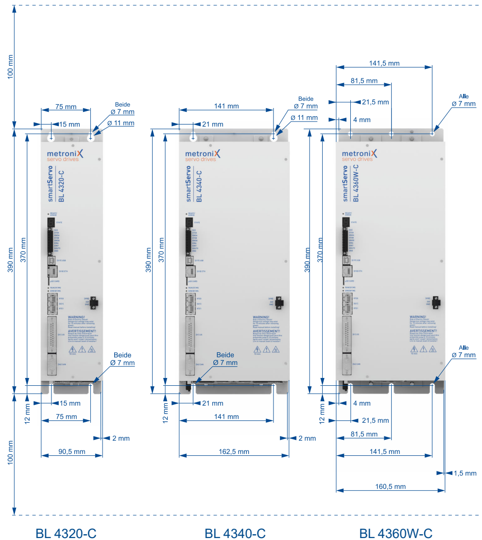
Abbildung 9: Maße und Einbaufreiraum BL 4320-C...BL 4360W-C
