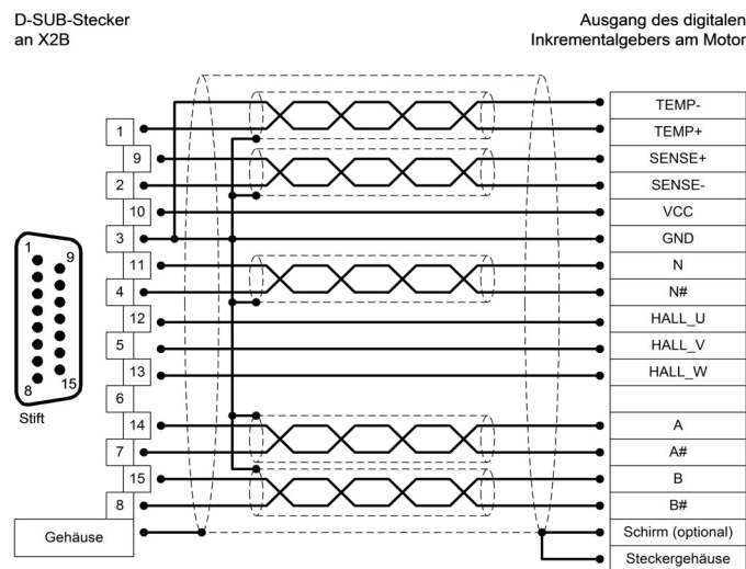
Abbildung 28: Steckerbelegung „Digitale Inkrementalgeber (RS422) [X2B]“
