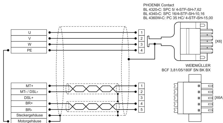
Abbildung 22: Steckerbelegung „Motor mit Motortemperatur-Sensor [X6]“
