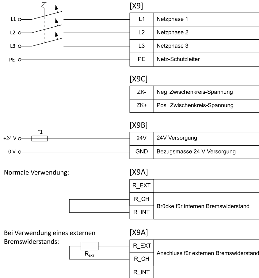
Abbildung 16: Anschluss eines BL 4320-C, BL 4340-C oder BL 4360W-C an die Versorgungsspannung [X9]
