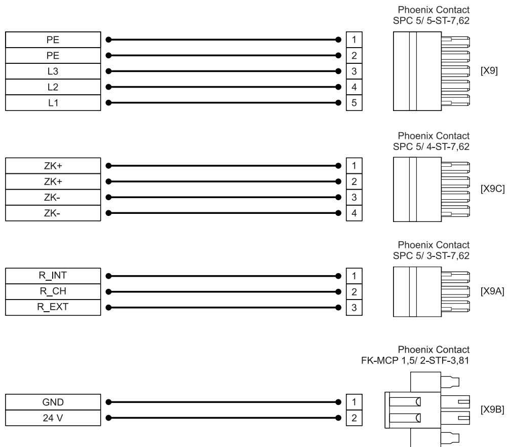
Abbildung 17: Steckerbelegung „Versorgungsspannung [X9], [X9A], [X9B], [X9C]“
