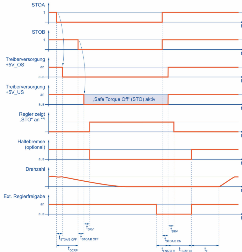
Abbildung 37: Zeitverhalten beim Aktivieren der Sicherheitsfunktion STO mit Wiederanlauf
