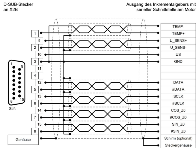
Abbildung 27: Steckerbelegung „Inkrementalgeber mit serieller Schnittstelle [X2B]“
