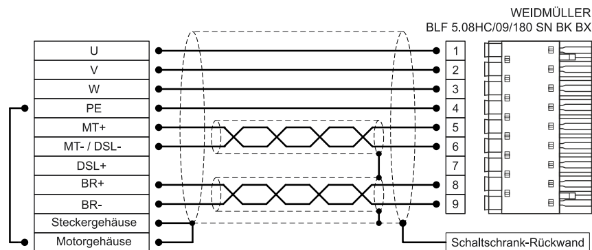
Abbildung 18: Steckerbelegung „Motor mit Motortemperatur-Sensor [X6]“
