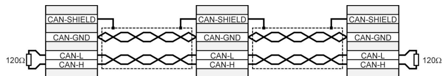
Abbildung 32: Verkabelungsbeispiel für CAN-Bus
