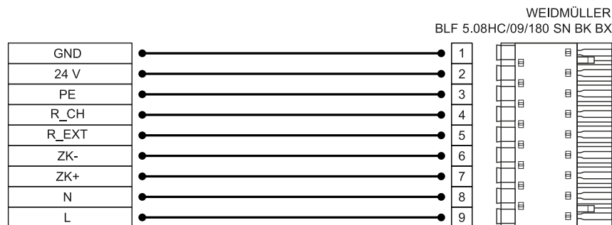
Abbildung 11: Steckerbelegung „Versorgungsspannung [X9]“
