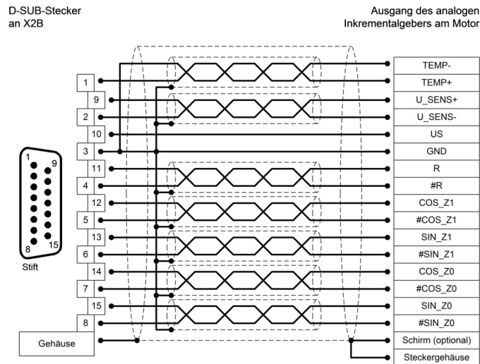
Abbildung 26: Steckerbelegung „Analoge Inkrementalgeber [X2B]“
