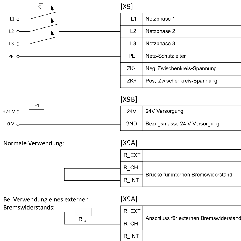
Abbildung 14: Anschluss eines BL 4304-C, BL 4308-C oder BL 4312-C an die Versorgungsspannung [X9]
