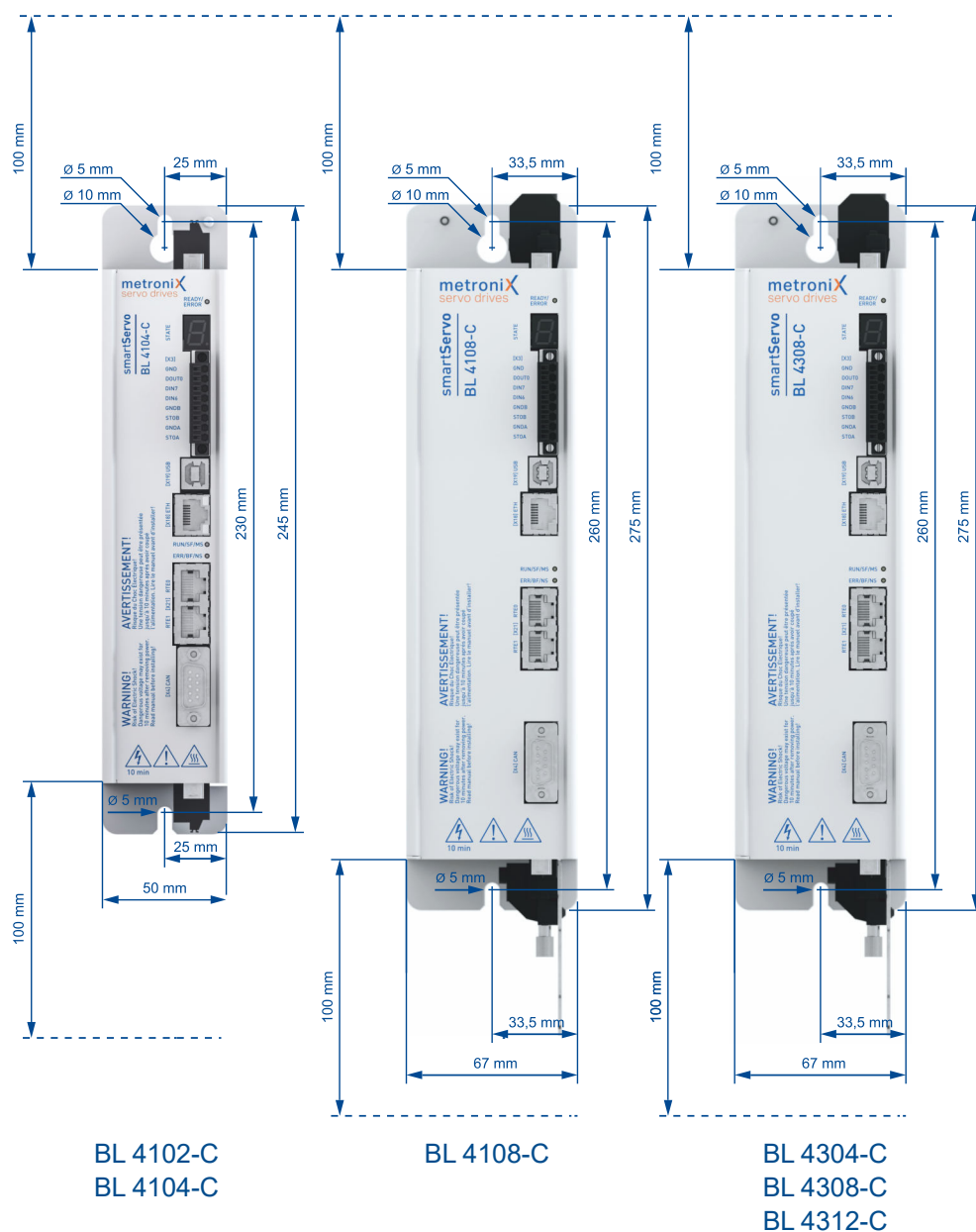
Abbildung 8: Maße und Einbaufreiraum BL 4102-C...BL 4312-C
